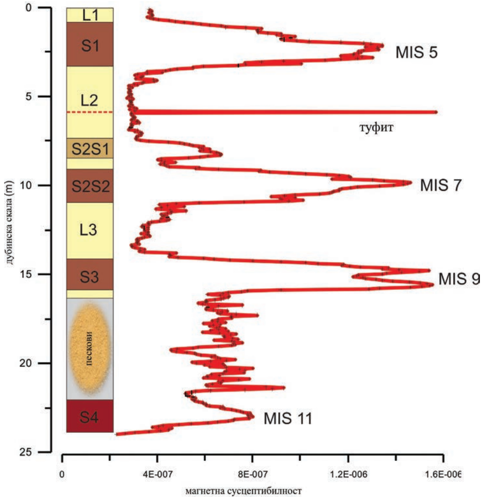
Слика 5. Сигнал масене магнетне суспенцибилности за заштићени профил у Земуну. Легенда: MIS – маринско-изотопски периоди; L – лес, S – палеоземљиште
