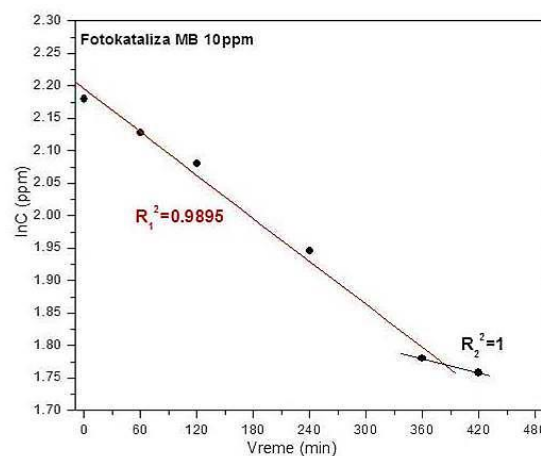
Slika 4.42. Promena koncentracije rastvora MB 10 ppm u funkciji vremena tokom procesa razgradnje u prisustvu čestica uzorka ZnO-13 SH.
