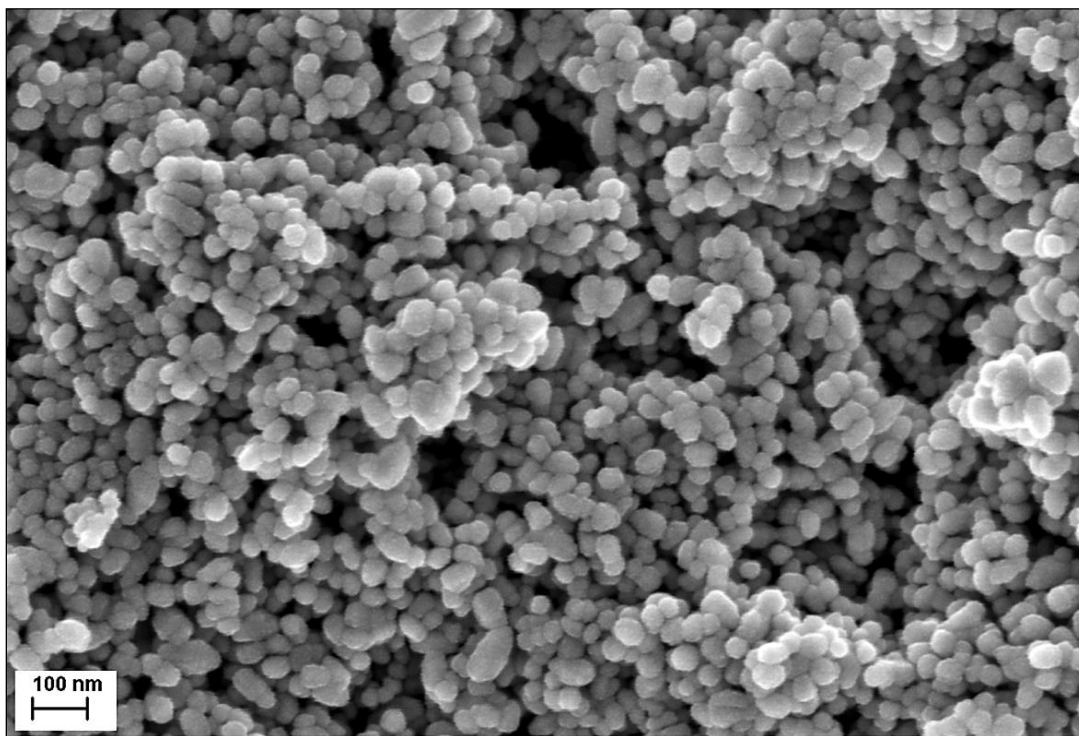
Slika 4.12. FE SEM fotografija praha ZnO-13.
