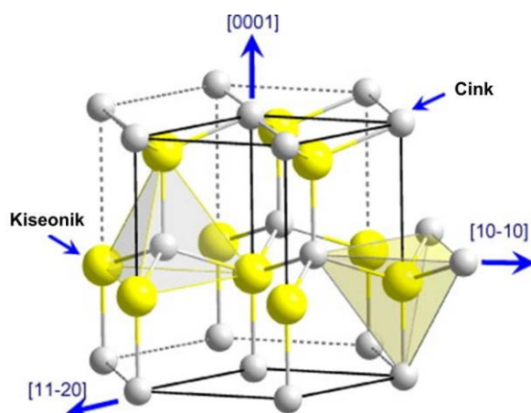
Slika 1.1. Šematski prikaz heksagonalne vrcitne strukture kristala ZnO^a .
