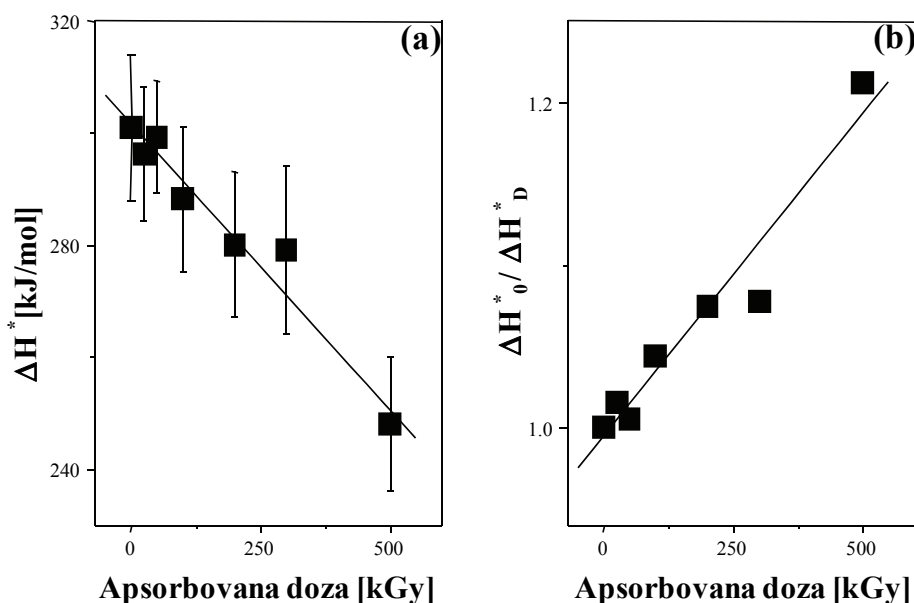
Slika 4. a) Prividna aktivaciona energija, \Delta H^* u funkciji od apsorbirane doze za PLLA uzorke; b) Odnos \Delta H^*_0 / \Delta H^*_D u funkciji apsorbirane doze; gde su \Delta H^*_0 i \Delta H^*_D aktivacione energije neozračenog i ozračenih uzoraka (do apsorbirane doze D ). Figure 4. a) Apparent activation energy, \Delta H^* as a function of absorbed dose for PLLA samples; b) \Delta H^*_0 / \Delta H^*_D ratio versus absorbed dose; where \Delta H^*_0 and \Delta H^*_D are activation energies of the unirradiated and irradiated samples (to absorbed dose D ), respectively.
