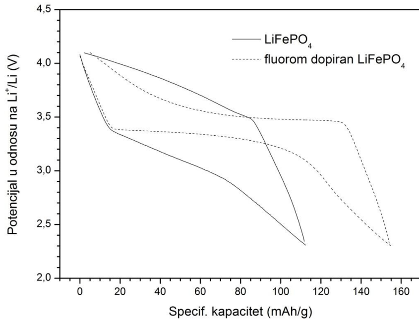
Slika 4.1.8 Elektrohemijski profil punjenja-pražnjenja pri brzini C/5 za uzorke LiFePO 4 i fluorom dopiranog LiFePO 4 na sobnoj temperaturi. Maseni odnos pri izradi elektroda bio je m_a:m_{cb}:m_{pvdF}=50:40:10 .
