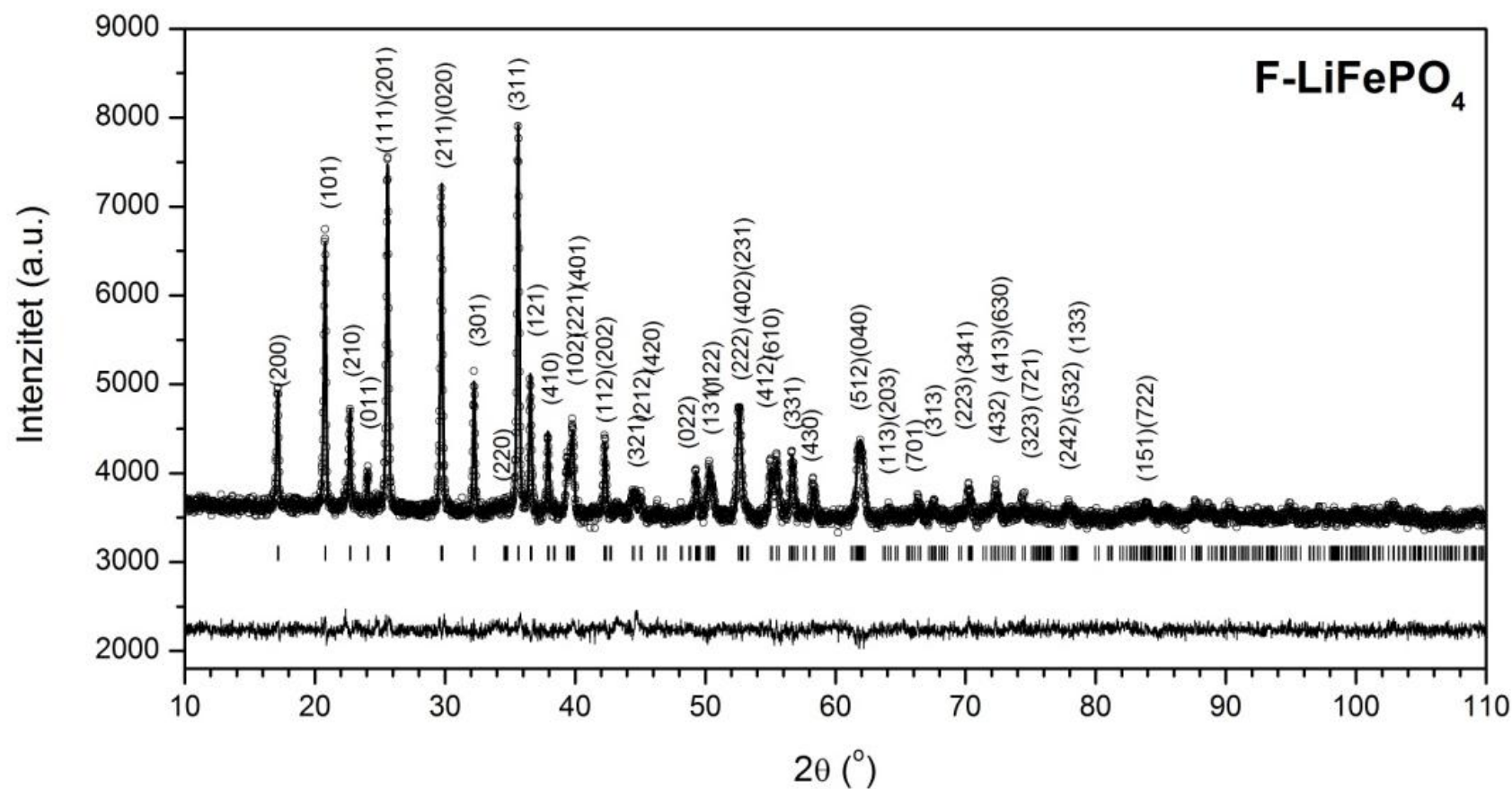
Slika 4.1.5 Grafički prikaz rezultata Ritveldovog utajčnjavanja strukture uzorka fluorom dopiranog LiFePO 4 (F-LiFePO 4 ). Tačkama (o) su prikazane eksperimentalne vrednosti, a punom linijom računate; na dnu je prikazana razlika između eksperimentalnog i izračunatog profila, a vertikalnim crticama označene su moguće pozicije Bragovih maksimuma. Glavni difrakcioni maksimumi označeni su Milerovim indeksima.
