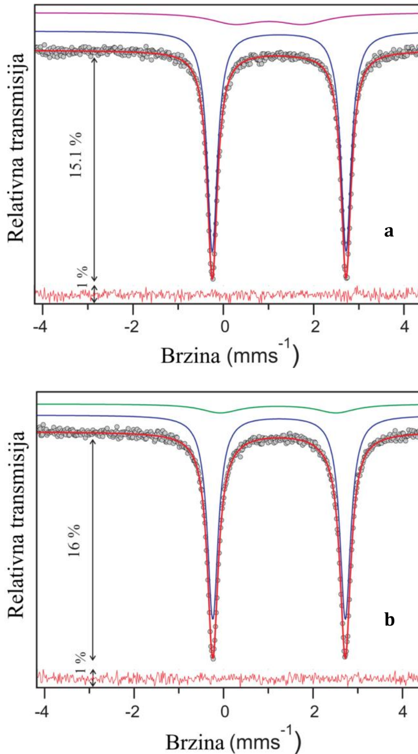
Slika 4.1.5 NGR spektri 57 Fe u uzorku LiFePO 4 (a) i fluorom dopiranom LiFePO 4 (b) na sobnoj temperaturi. Eksperimentalne tačke su prikazane kružićima, dok su teorijske krive prikazane punom linijom crvene boje. Iznad su prikazane teorijske krive podspektara: plava – dublet A, ljubičasta – dublet B, zelena – dublet C. Crvena linija u donjem delu predstavlja razliku između eksperimentalne i teorijske krive.
