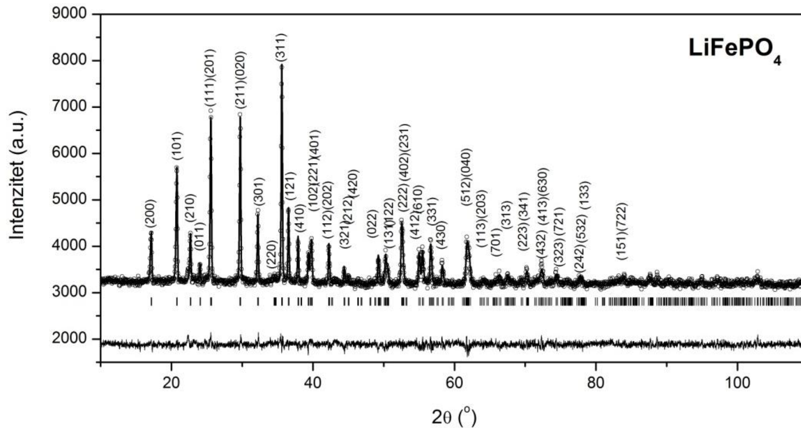
Slika 4.1.4 Grafički prikaz rezultata Ritveldovog utajčavanja strukture uzorka \text{LiFePO}_4 . Tačkama ( \circ ) su prikazane eksperimentalne vrednosti, a punom linijom računate; na dnu je prikazana razlika između eksperimentalnog i izračunatog profila, a vertikalnim crticama označene su moguće pozicije Bragovih maksimuma. Glavni difrakcioni maksimumi označeni su Milerovim indeksima.
